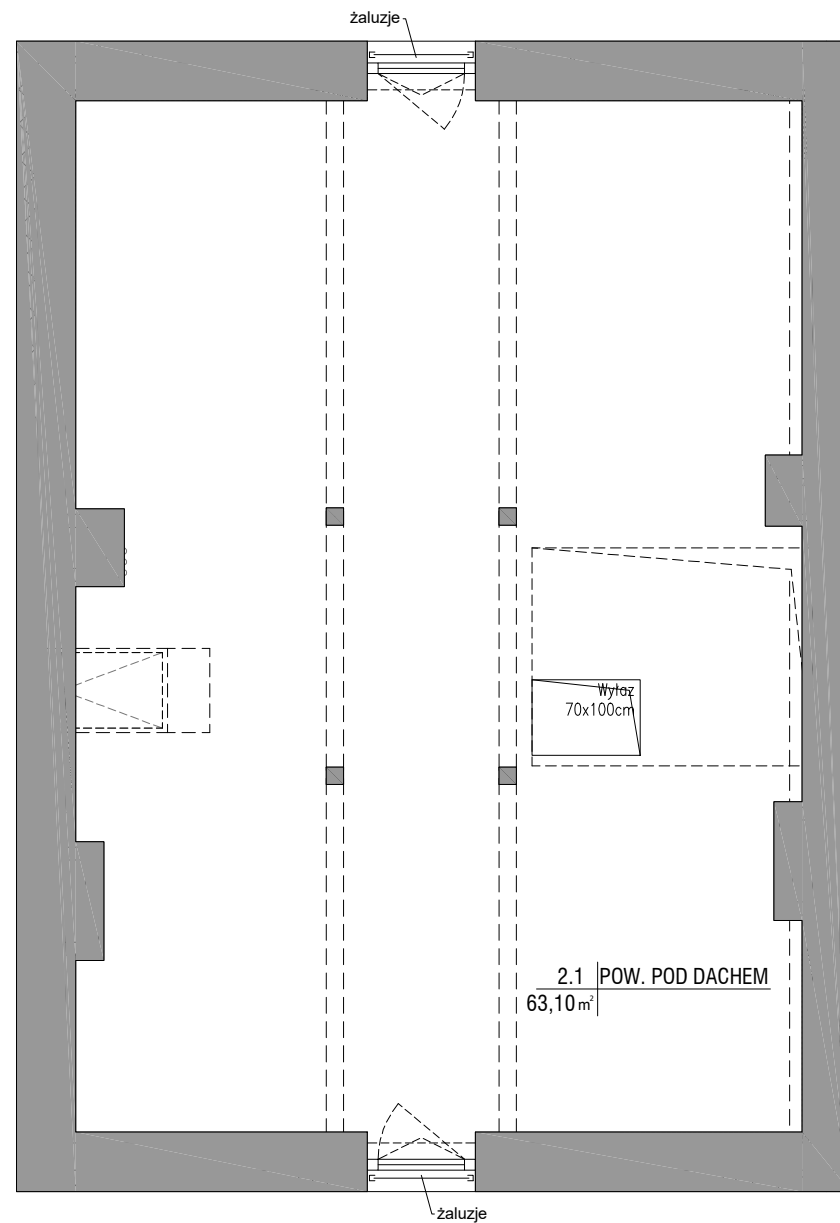
RZUT
