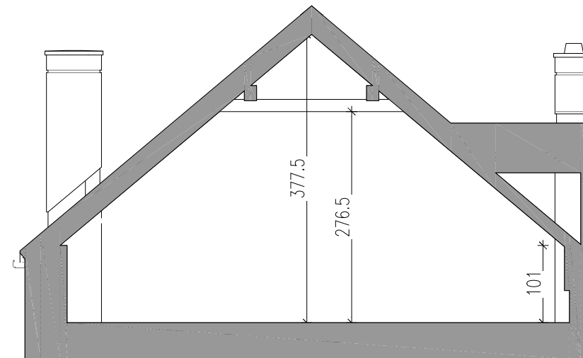
PRZEKRÓJ A-A
