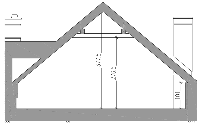
PRZEKRÓJ A-A
