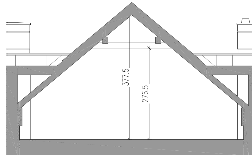
PRZEKRÓJ A-A
