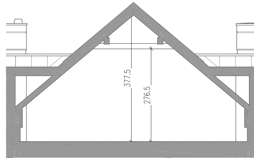
PRZEKRÓJ A-A
